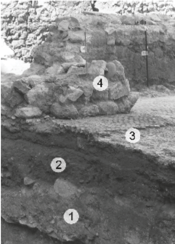
FIGURA 5. Detalle de la preparación constructiva del mosaico de edificio termal del s. III (Macías 2004). 1. Cimentación edificio portuario anterior; 2. relleno de abandono del edificio portuario; 3. mosaico con lecho de mortero (1-2 cms); 4. muro compartimentación doméstico de época visigoda. Foto: Codex / J. M. Macías.
