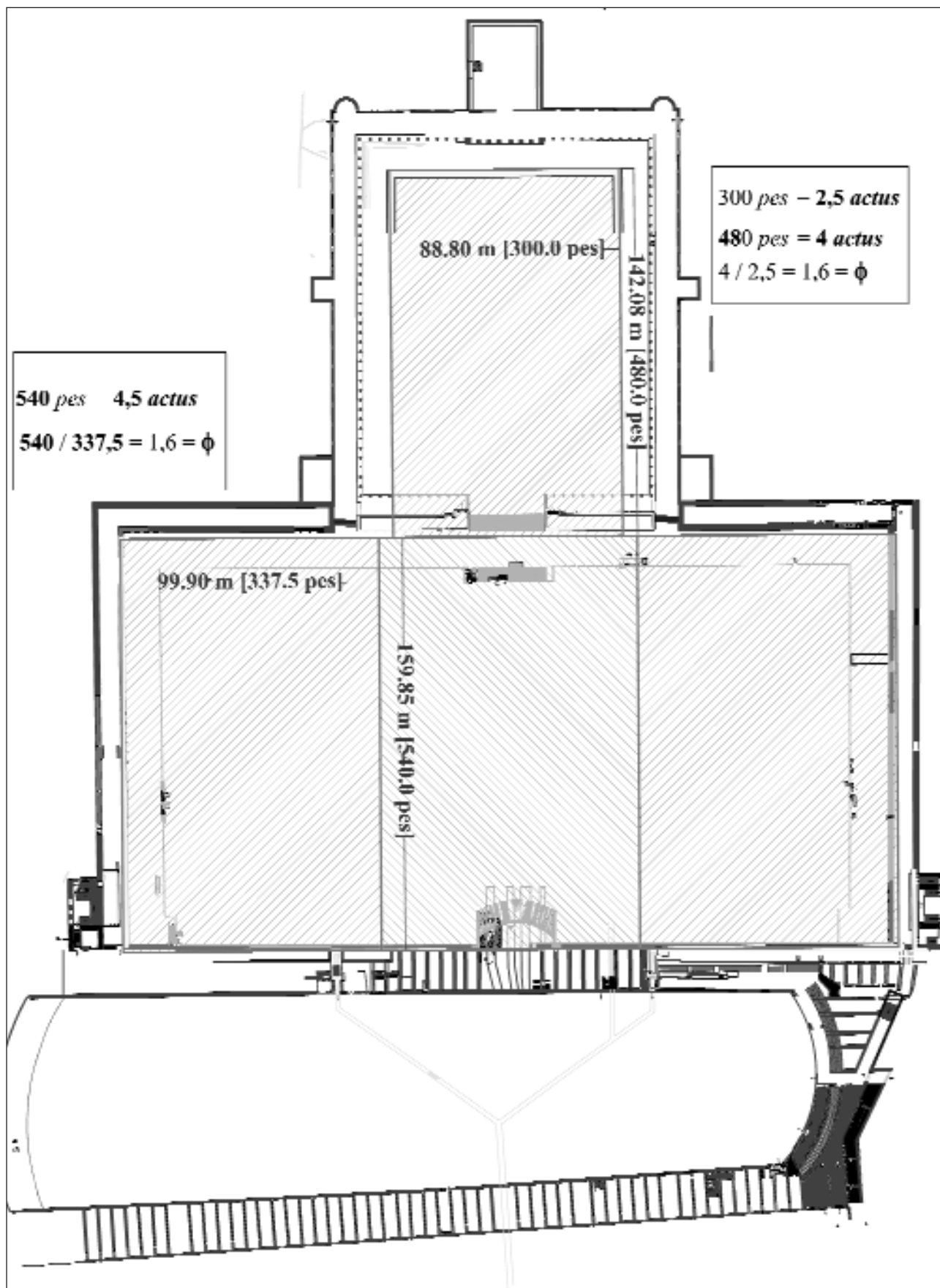
Fig. 26: Esquematització geomètrica del primer projecte de transformació urbanística de la Part Alta.
