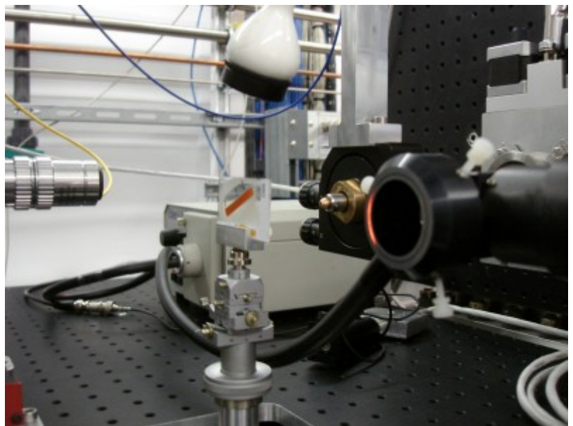
Muntatge de la làmina sobre un portamostra per fer les mesures en la fase d'anàlisi al Sincrotró ALBA. (Foto: Roberta Di Febo)
