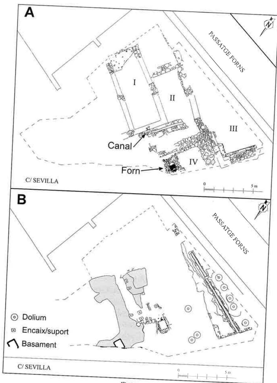
Figura 4: A. Planta fase republicana, forn de terrissa. B. Planta centre producció vinícola del s. III dC.
