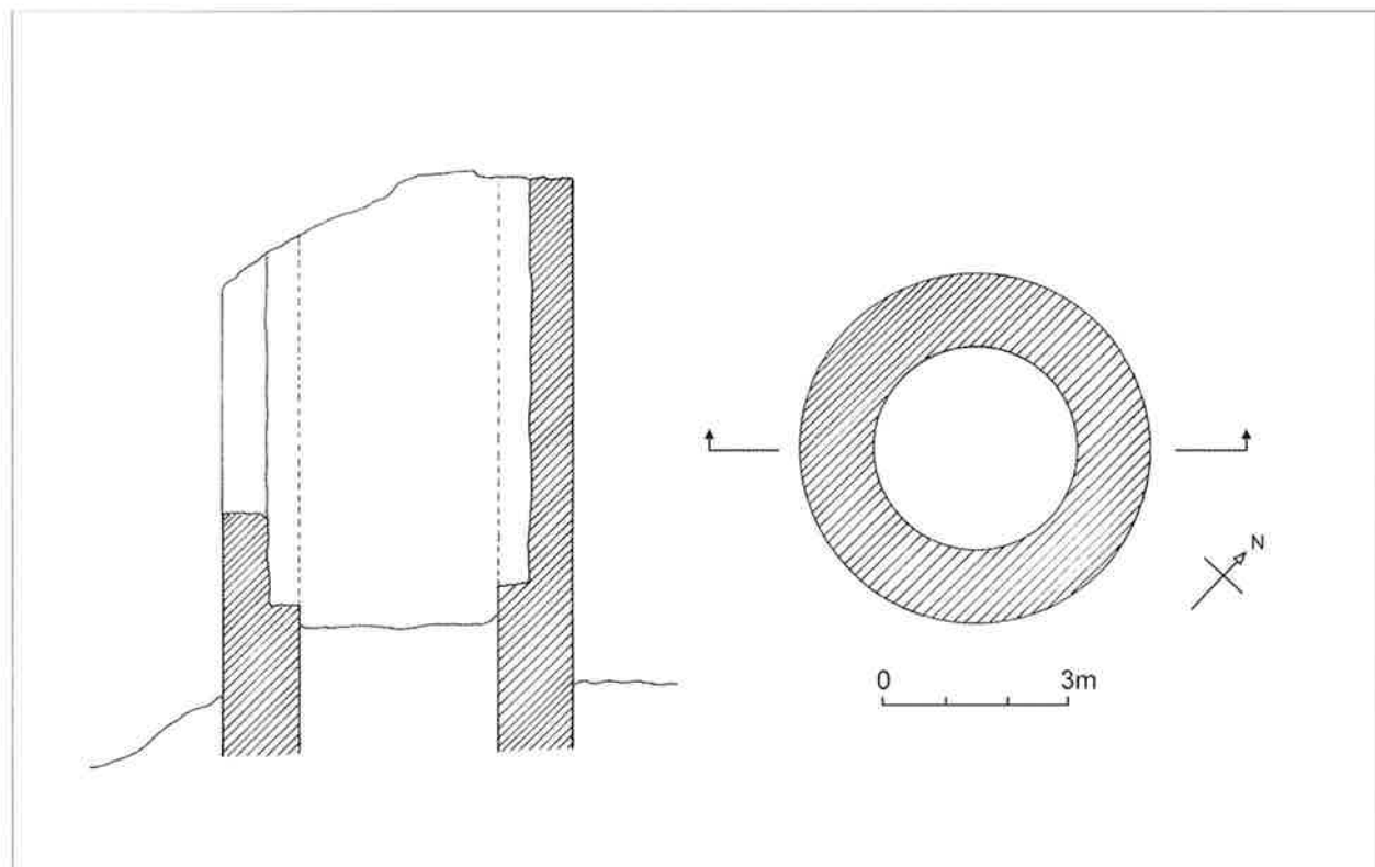
Figura 3: secció i planta de la torre. (J. Zaragoza).
