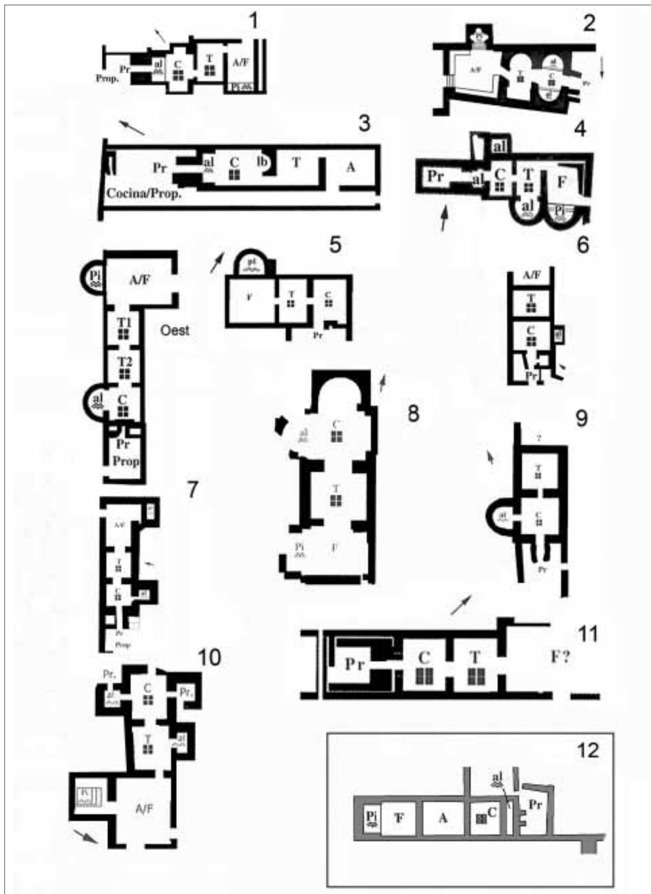
FIGURA 4. Paral·lels de banys similars d' Hispania (reelaboració a partir de García-Entero 2005): 1. Casa del Mosaico del Oso; 2. Casa de los Mármoles; 3. Casa 2B d'Empúries; 4. Nossa Senhora da Tourega Sur; 5. Torre de Palma 1; 6. C. Raposeira; 7. Illeta; 8. El Cogoll; 9. Font del Vilar; 10. Pla de Palol; 11. Camp de la Torre; 12. La Llosa.
