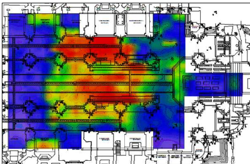
Mapa preliminar de resistivitat elèctrica a sota el paviment de la catedral obtinguda per interpolació de tots els perfils 2D de tomografia elèctrica.
