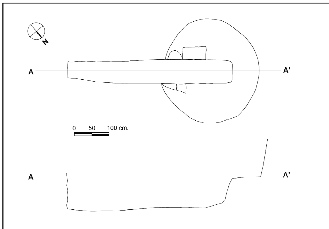
Forn. Planta i alçat.
