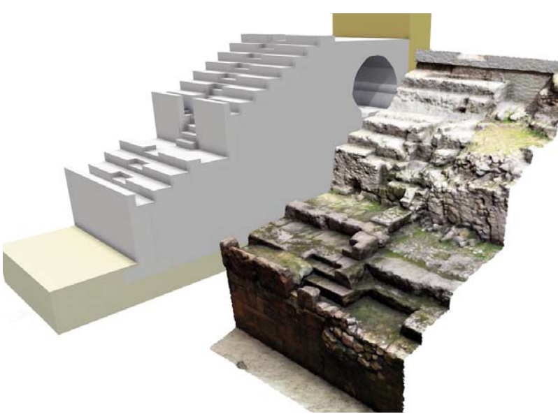
Esquema dels mòduls que integren el prototipus
