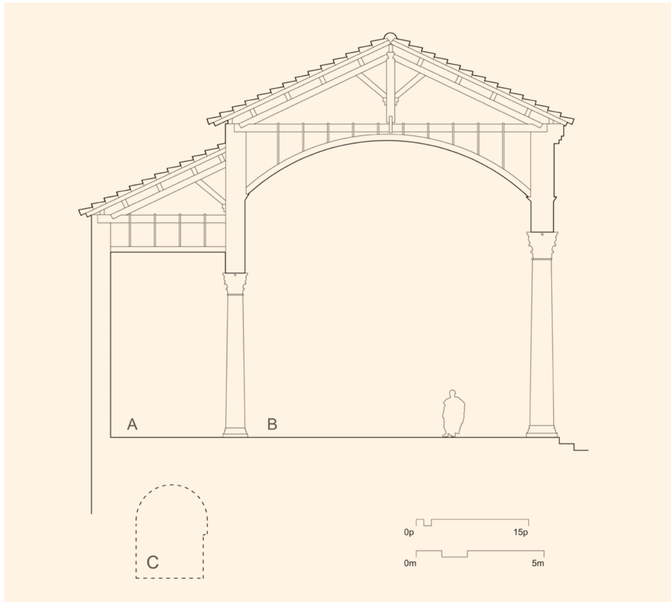
15 Exedra oriental de l'àrea sacra al Museu Bíblic (A), pòrtics perimetrals de l'àrea sacra (B) i possible volta de sustentació de l'exedra romana reutilitzada, en un moment indeterminat, com a cisterna (C). El mur de tancament d'aquesta volta pel sector nord-oriental correspon al mur de pseudo opus vitattum conservat a la seu del Consell Comarcal del Tarragonès (dibuix de l'arquitecta Elisenda Rosàs Tosas)
