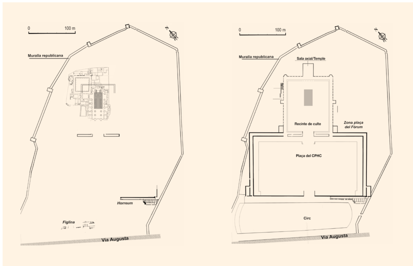
9 Planta comparativa dels dos projectes del recinte de culte (planimetria base, Macias et al. 2007b)
