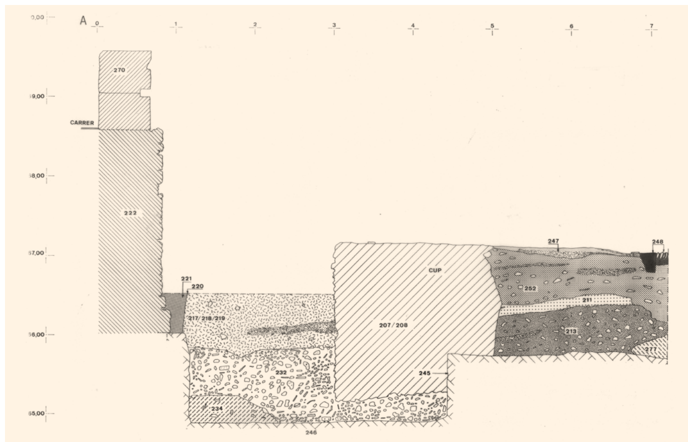
11 Secció i vista de les estructures de fonamentació de l'Antic Hospital, construïdes en el límit i, a la vegada, a l'interior de la trinxera constructiva del primer projecte de tèmenos (foto: TED'A)
