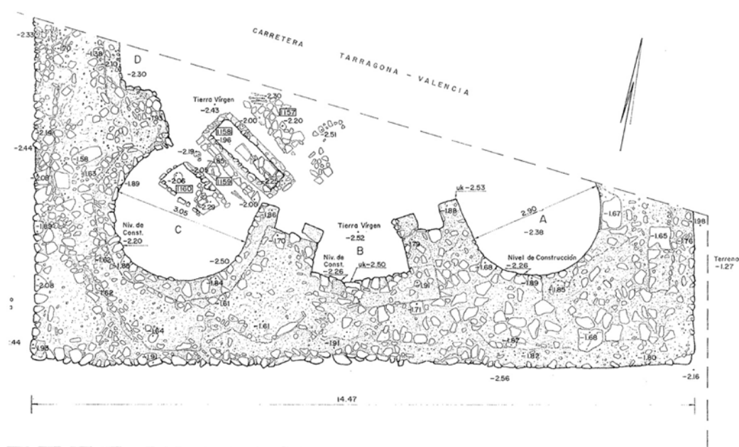
Figura 6 Mausoleu tardo antic de Tàrraco (gravat del segle XIX i planta de Hauschild 1975).
