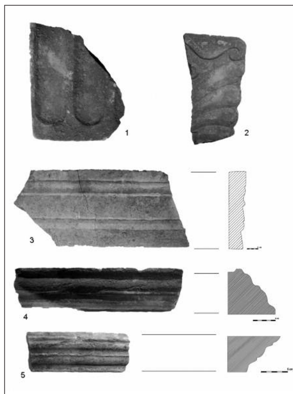
Fig. 2. Selección de elementos del revestimiento arquitectónico. 1. Fragmento de fuste. 2. Fragmento de capitel. 3. Placa de arquitrabe. 4. Moldura de base. 5. Moldura de coronamiento.
