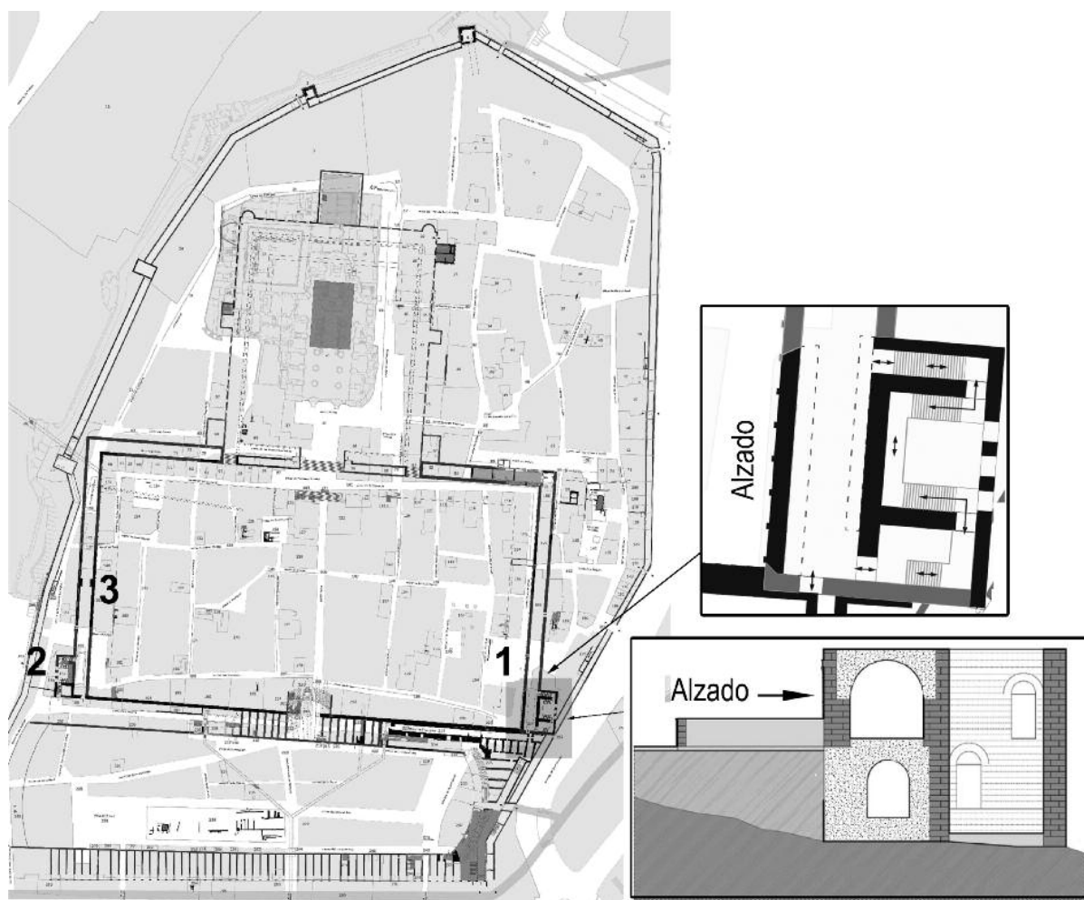
Fig. 1. Planta de la sede monumental del Concilium Prouvinciae Hispaniae Citerioris (Macias et al. 2007): 1, Torre del Pretorio; 2, Torre de la Antigua Audiencia.
