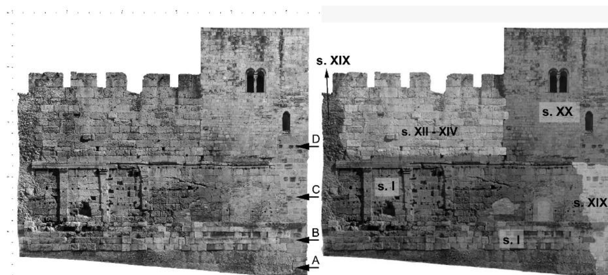
Fig. 3. Ortofoto del lienzo de pilastras (original y texturizado por fases edilicias): A, cimentación en opus caementicium ; B, cimentación en opus quadratum ; C, muro decorado con pilastras; D, restauraciones posteriores.
