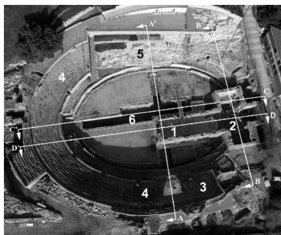
Fig. 1. Imagen aérea del complejo e indicaciones de la figura 3 (Archivo Desdelt-Ayuntamiento Tarragona-ICAC): 1, cimentación Basílica visigoda; 2, Iglesia medieval; 3, gradería original; 4, gradería reconstruida; 5, gradería excavada en la roca; 6, fossae .
