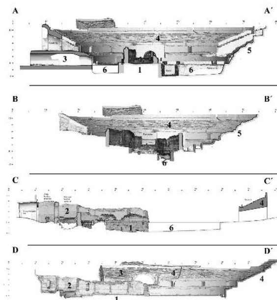
Fig. 3. Secciones, alzados y proyecciones obtenidos del escáner láser: 1, cimentación Basilica visigoda; 2, Iglesia medieval; 3, gradería original; 4, gradería reconstruida; 5, gradería excavada en la roca; 6, fossae .
