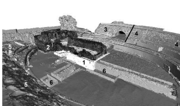
Fig. 2. Vista general obtenida a partir de la información del escáner láser: 1, cimentación Basilica visigoda; 2, Iglesia medieval; 3, gradería original; 4, gradería reconstruida; 5, gradería excavada en la roca; 6, fossae .
