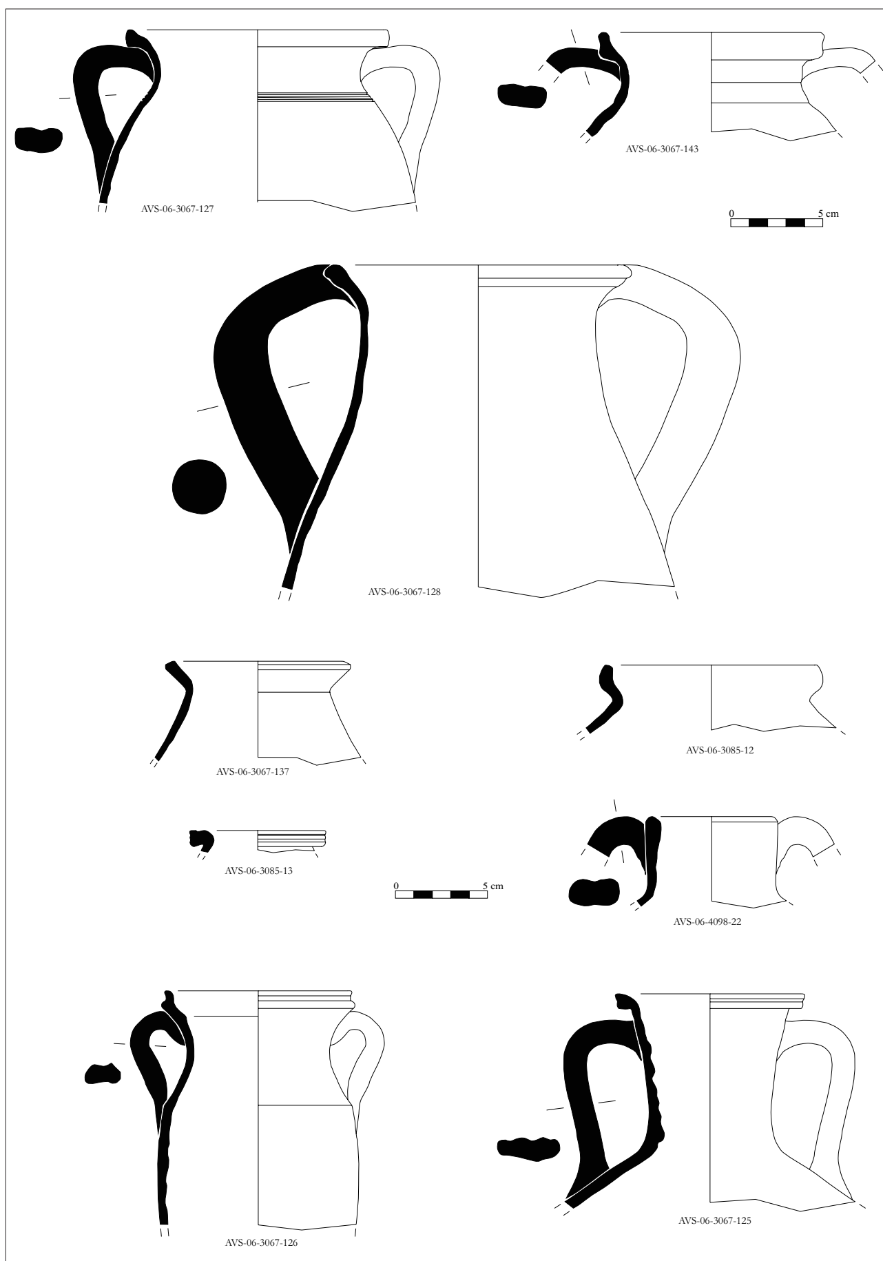
FIGURA 14. Gerres produïdes al Vila-sec.
