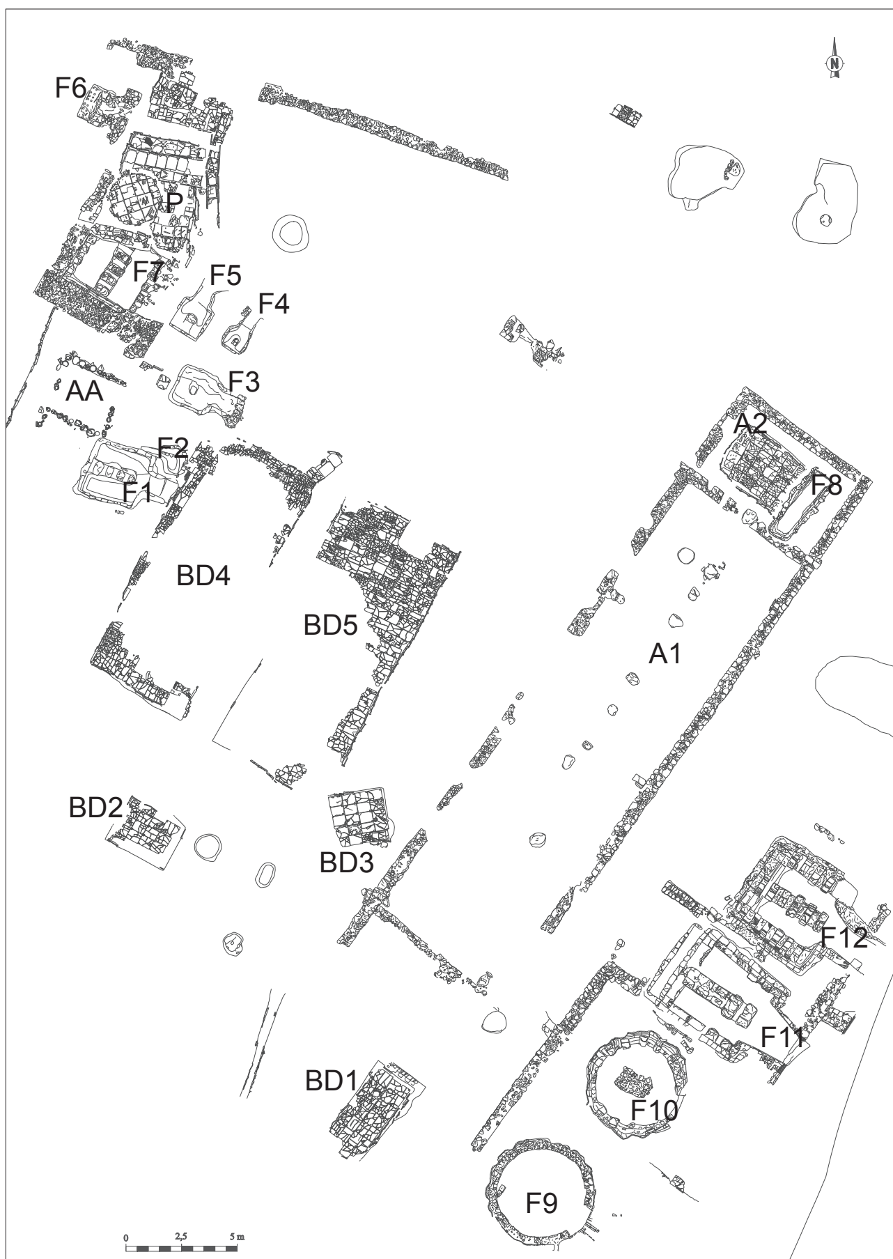
FIGURA 1. Planta general de la bòbila del Vila-sec.
