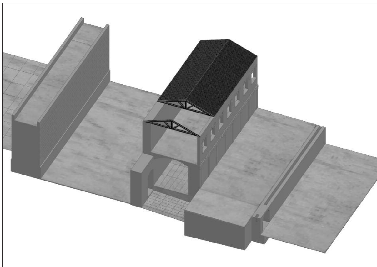
Fig. 3. Perspectiva S-N de la restitución hipotética de la gran tribuna elevada, cerrada por el muro de pilastras, en relación con el criptopórtico y la muralla (M. Díaz, M. Schillaci).
