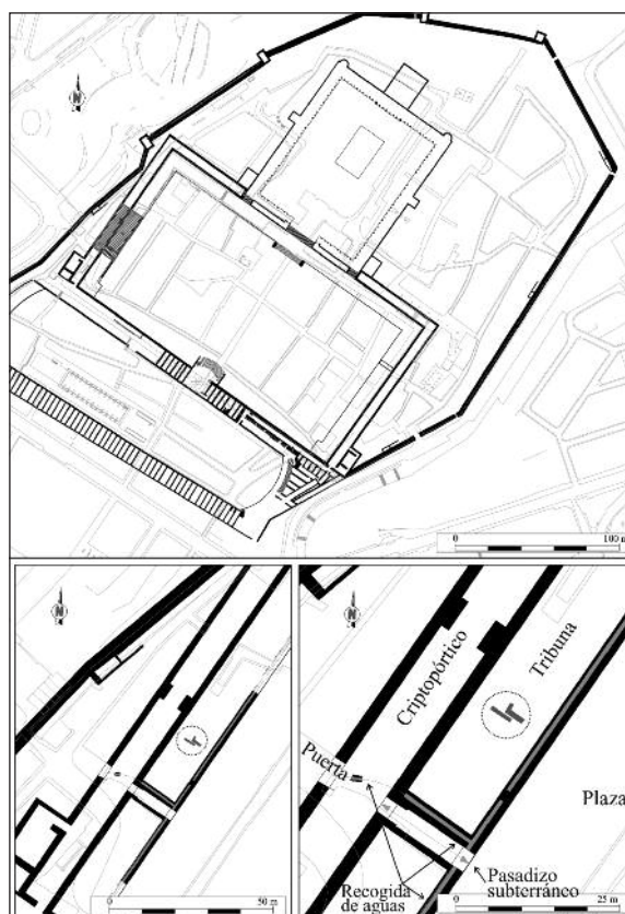
Fig. 1. Arriba: planta de situación del área intervenida. Debajo: detalle de las estructuras de la plaza de representación documentadas en nuestra excavación, con la zona central de la tribuna reocupada por estructuras en época tardoantigua –enmarcadas– (Archivo Codex-Arqueología i Patrimoni).
