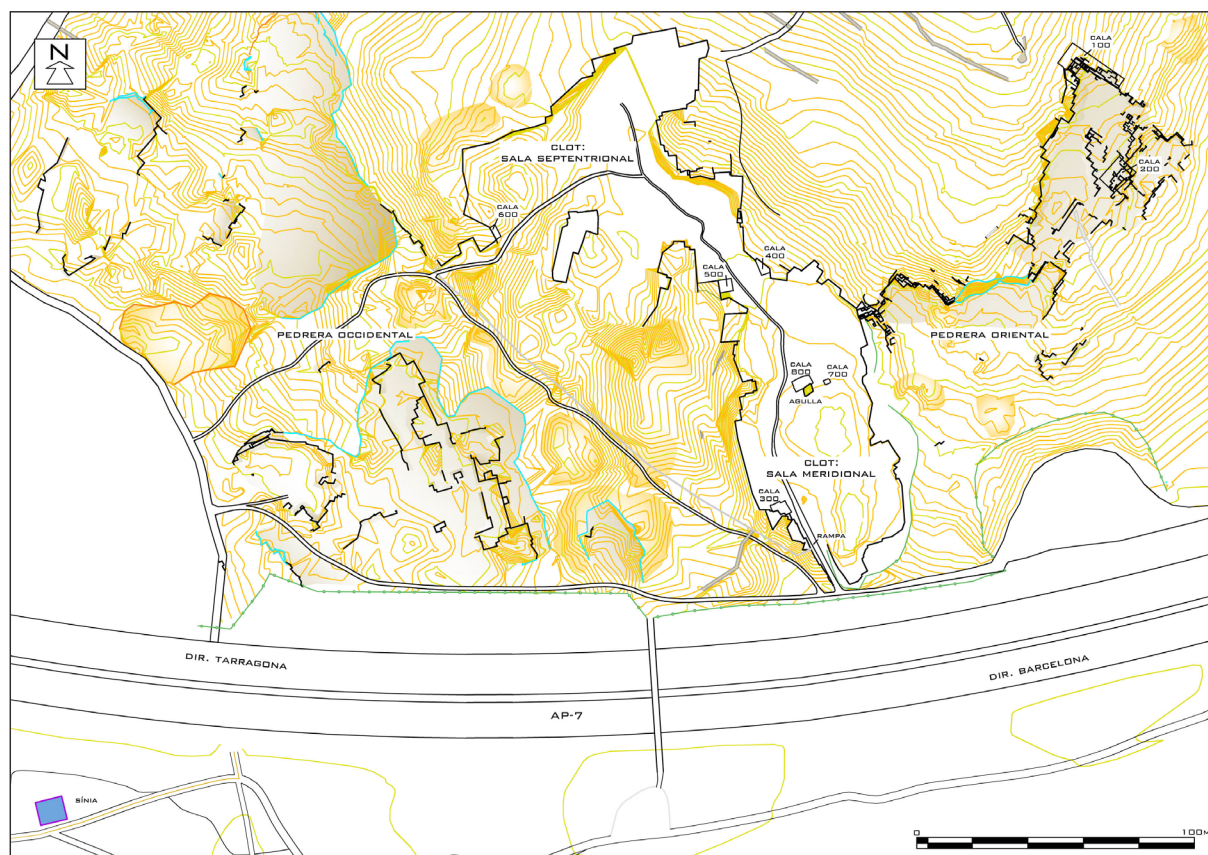
Figura 1. Planta general del Mèdol (Unitat de Documentació Gràfica ICAC)
