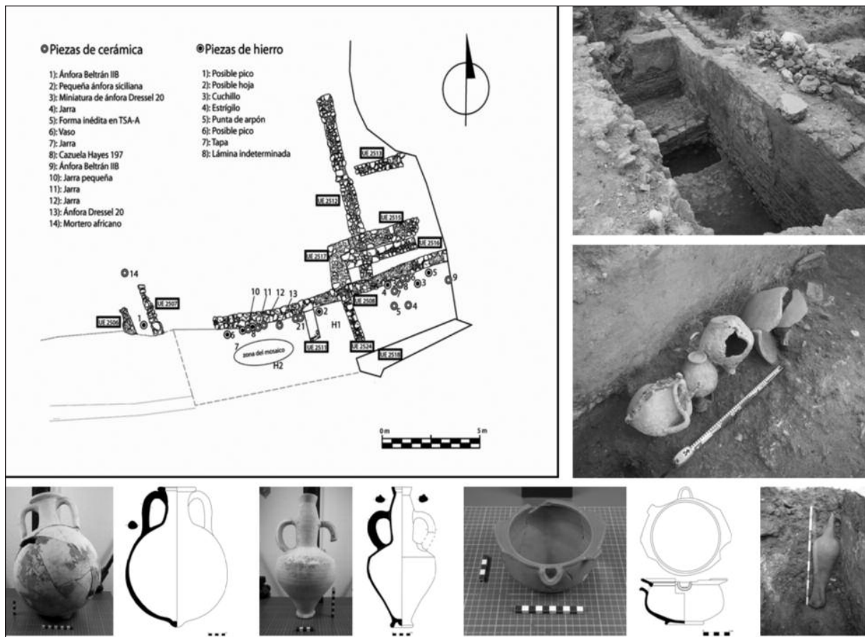
Fig. 2. Planta de las estructuras romanas halladas en Sant Felip Neri, con la situación de los hallazgos muebles.
