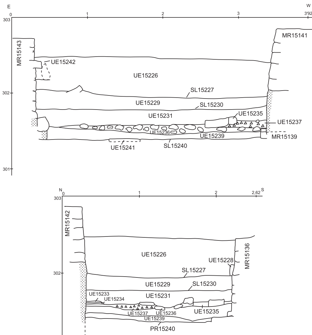
Fig. 8. Seccions sector 64
