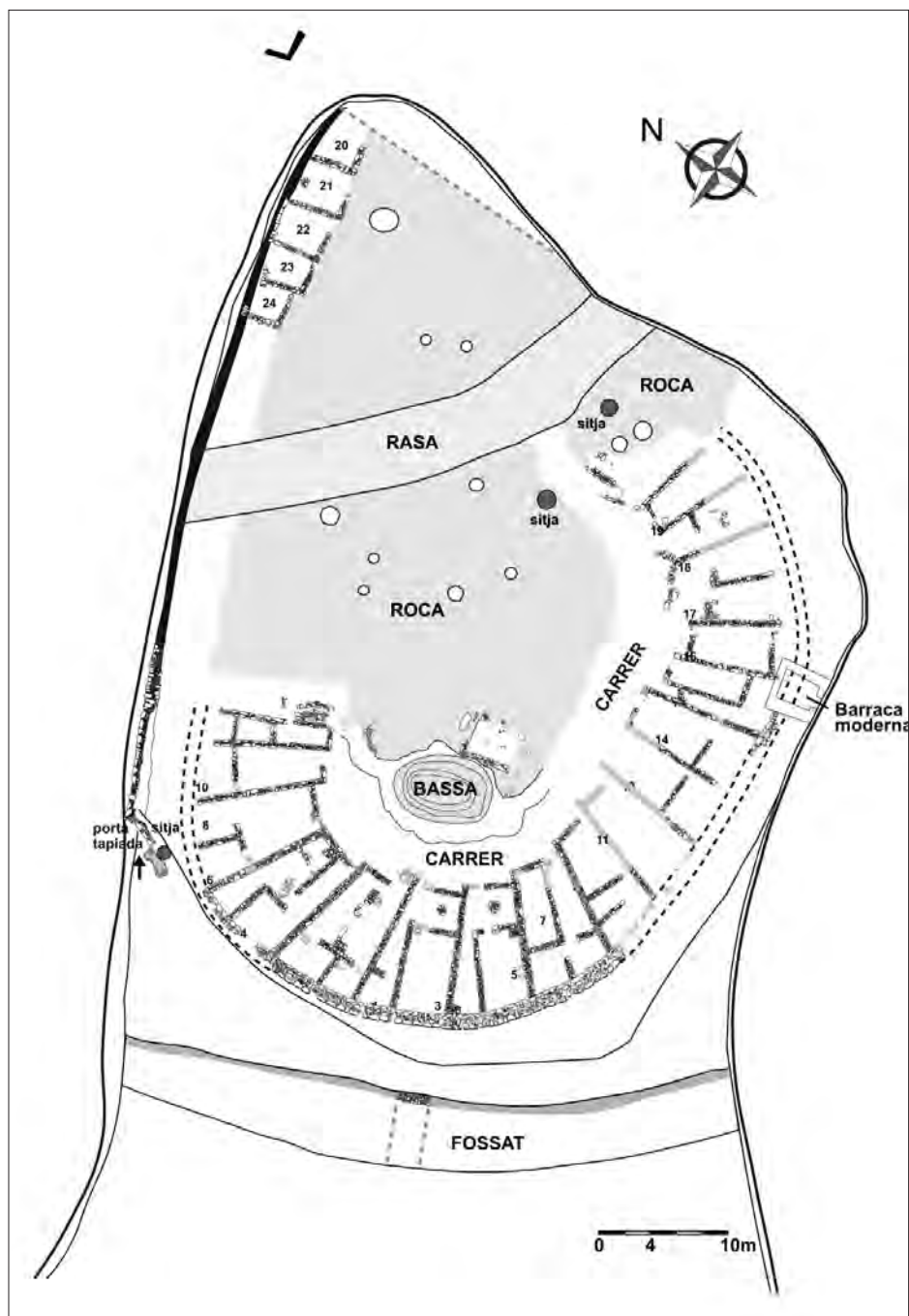
Figura 4. Planta general de l'assentament d'Estincells (segons Asensio et alii 2009: 27, figura 3).
