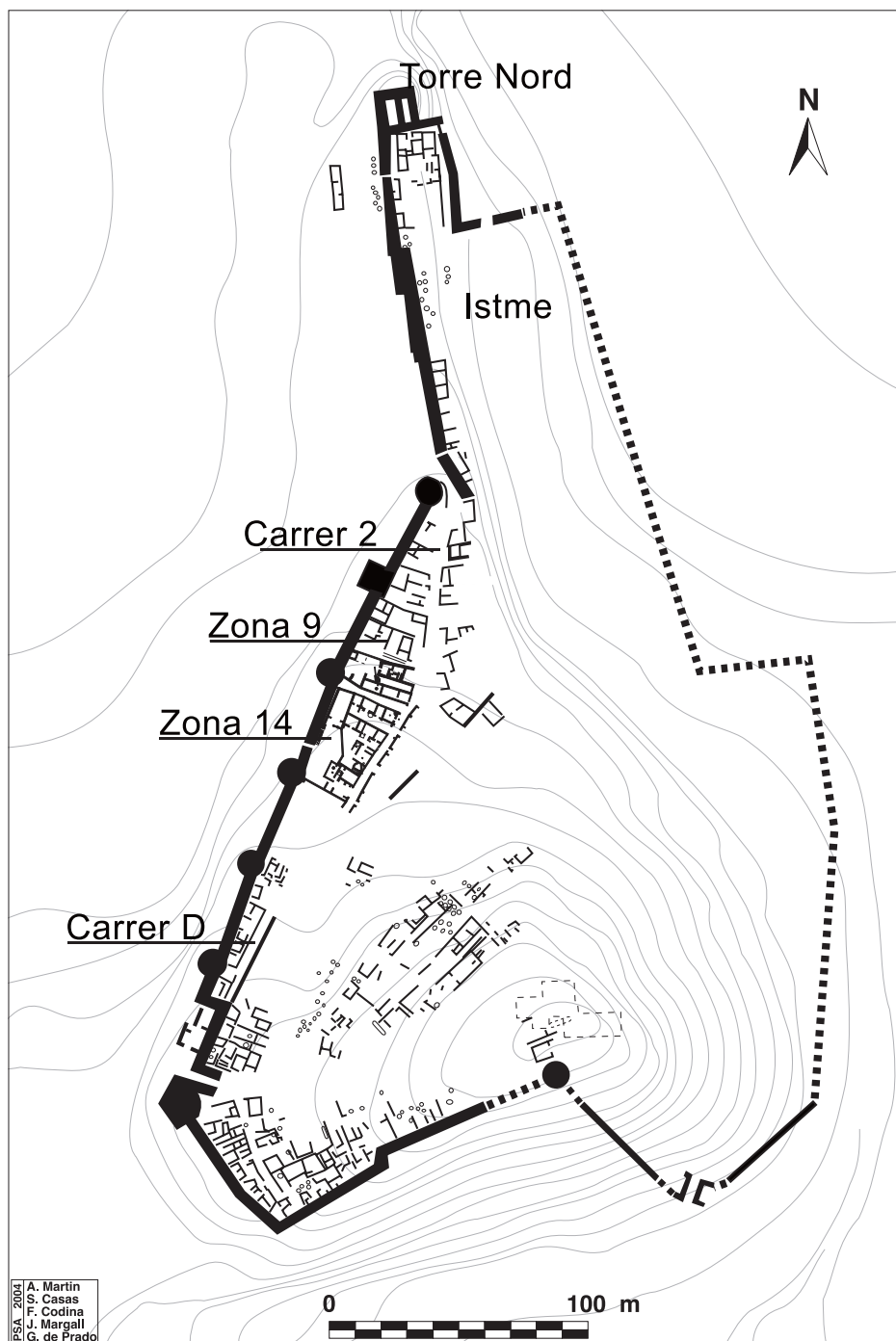
Figura 9. Planta general del Puig de Sant Andreu d'Ullastret (cedida per Aurora Martín).
